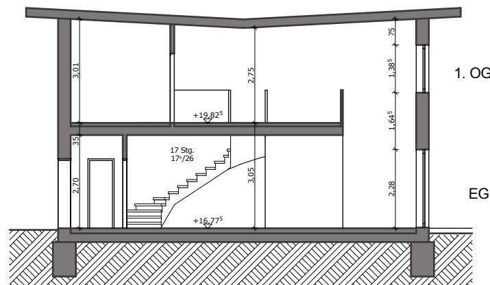
Schnitt Haus 3
