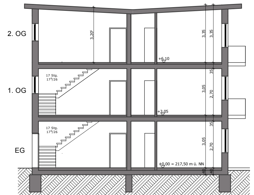
Schnitt Haus 2
