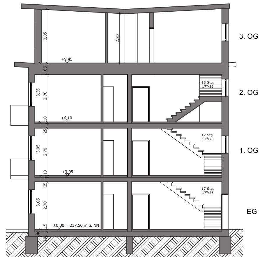
Schnitt Haus 1
